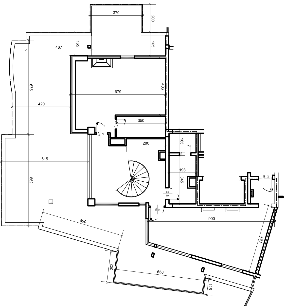
PLANIMETRIA E APARTAMENTIT 49 , KATI 9, (KUOTA +30.55) SHKALLA 1:150
